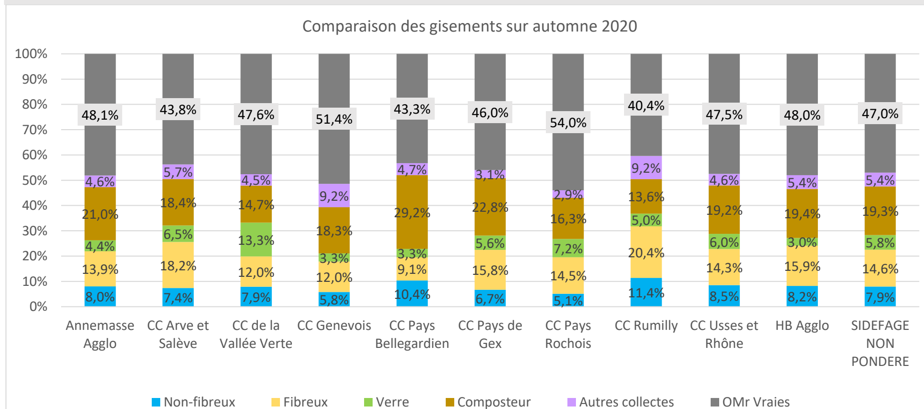
Graphique 57: Composition comparée des OMR des collectivités du SIDEFAGE A2020
